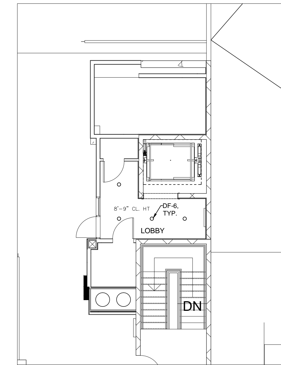
SE ELEV SCALE: 1/8" = 1'-0"
