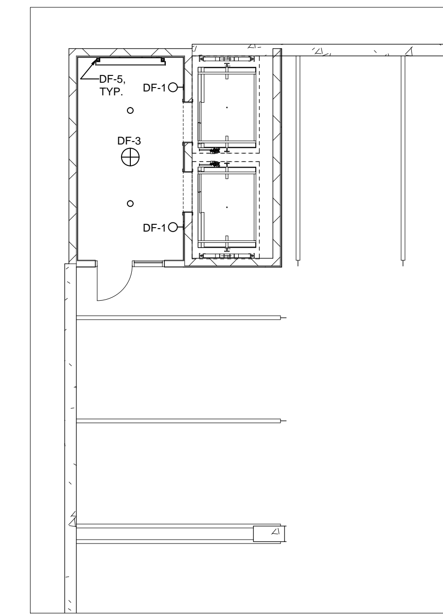
NW ELEV. SCALE: 1/8" = 1'-0"
