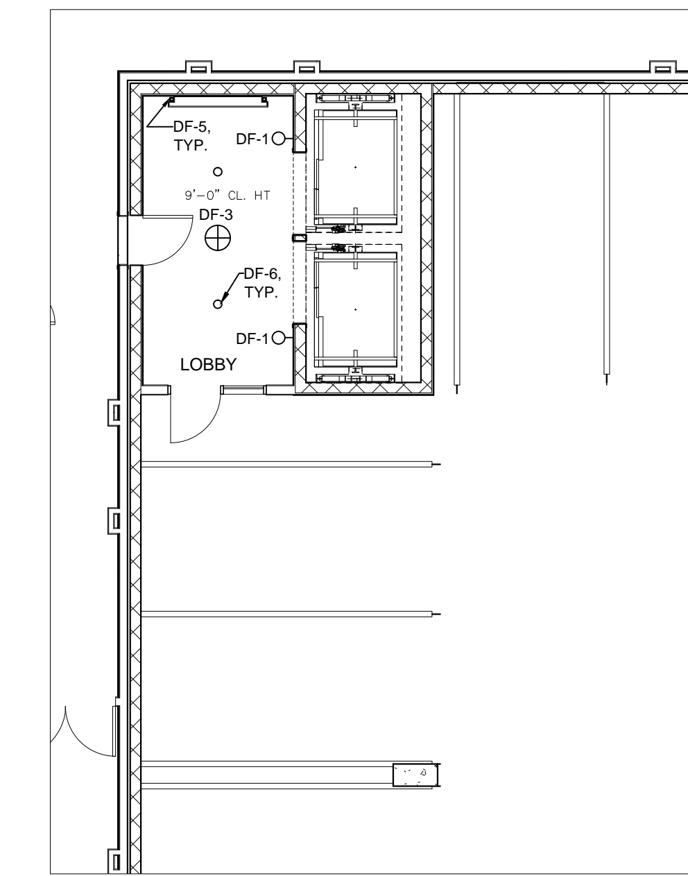
NW ELEV. SCALE: 1/8" = 1'-0"
