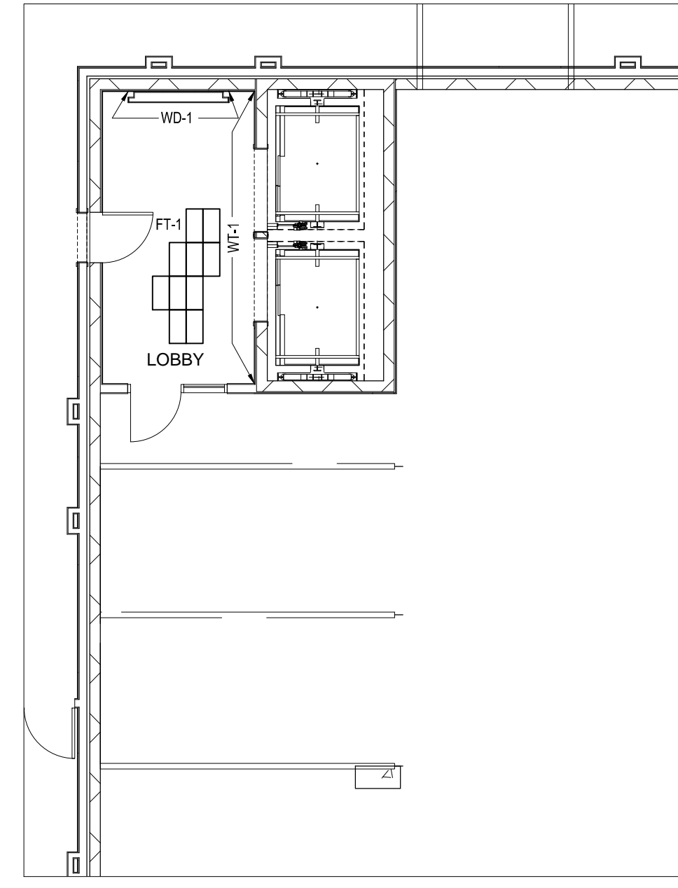
NW ELEV. SCALE: 1/8" = 1'-0"
