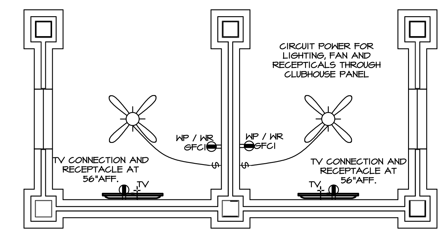
CABANA POWER N.T.S.
